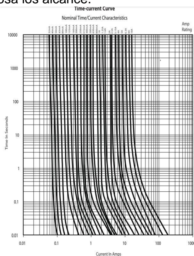
Grafica 1. Curvas tiempo-corriente de fusibles
